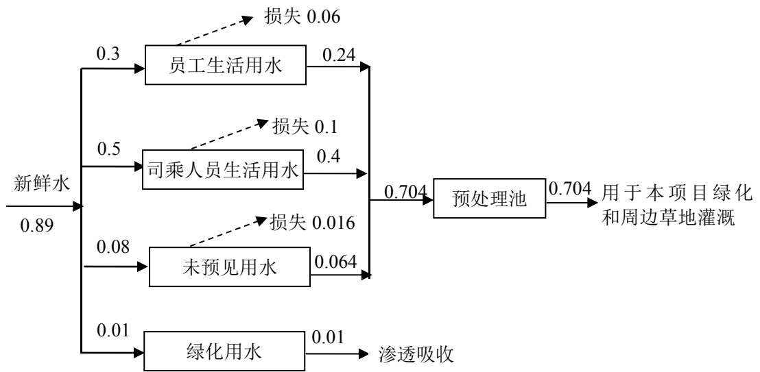
图 2-1 项目最大水量平衡见图 (m³/d)
